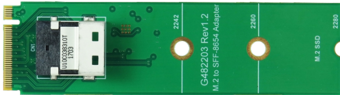
Top side
